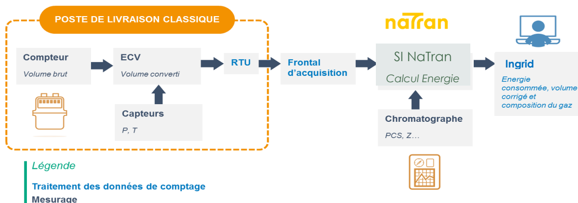
Figure 1 : Chaîne de comptage pour un poste de livraison classique
