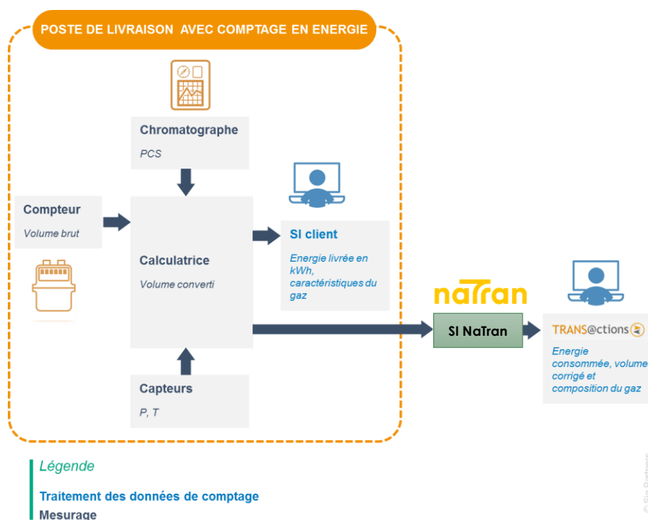
Figure 2 : Chaîne de comptage pour un poste de livraison avec comptage en énergie
