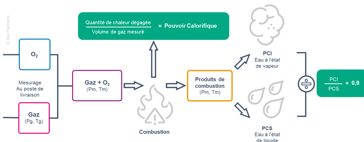
Figure 6 : Principe de détermination du PCS selon la norme NF EN ISO 6976-2005 4
